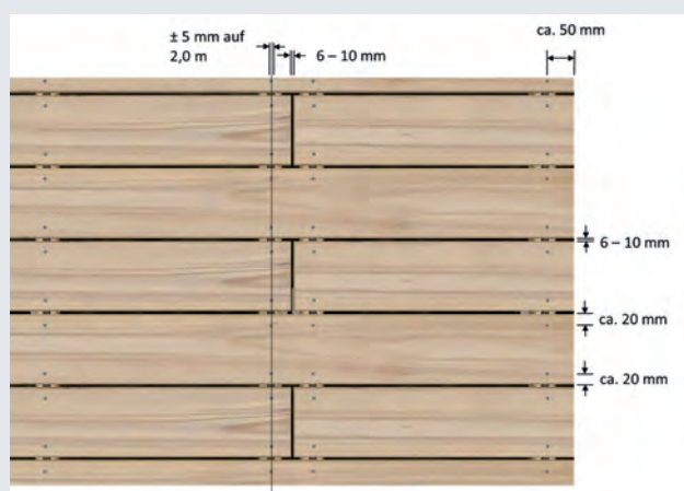
Abstände und Toleranzen von Fugen und Verschraubungen
