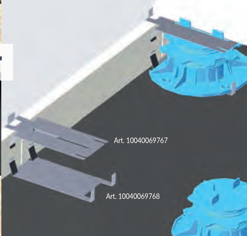
Abbildung 2: Montage mit Abschlussleiste
