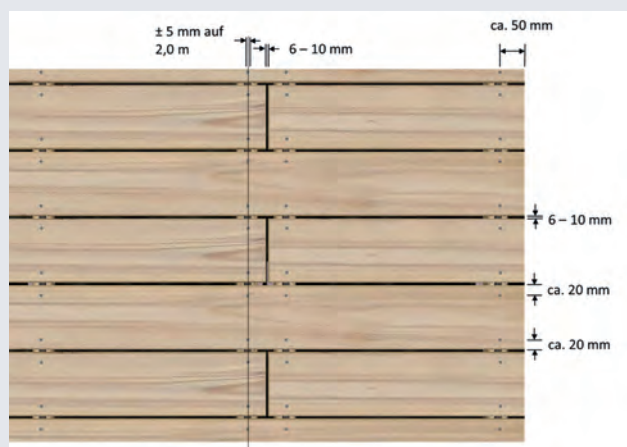
Abstände und Toleranzen von Fugen und Verschraubungen
